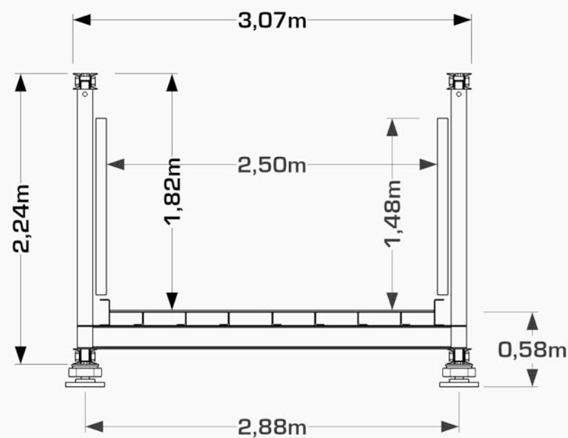
Vorderansicht
