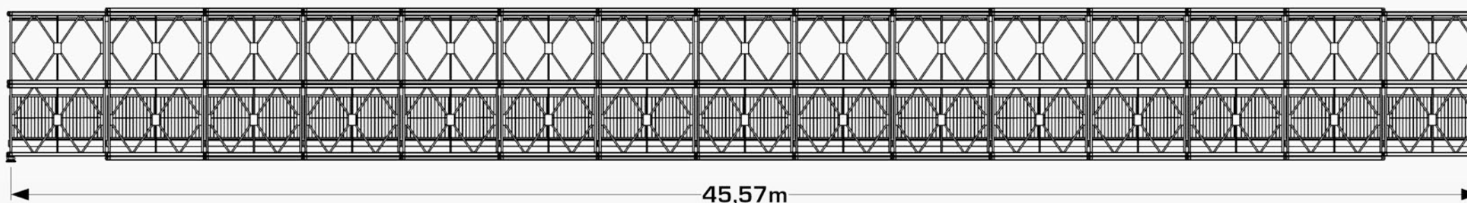
Seitenansicht
