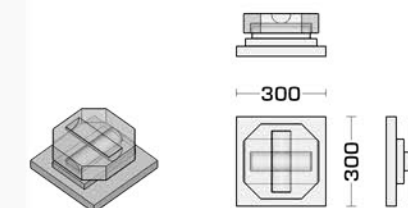
Detail: Lagerplatte
