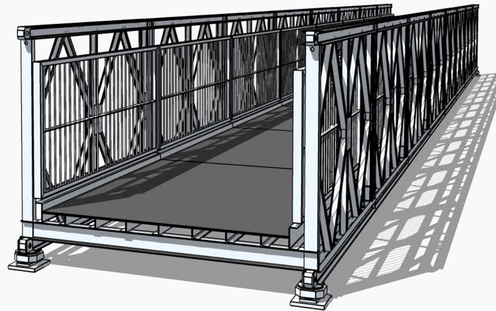
3D-Darstellung
