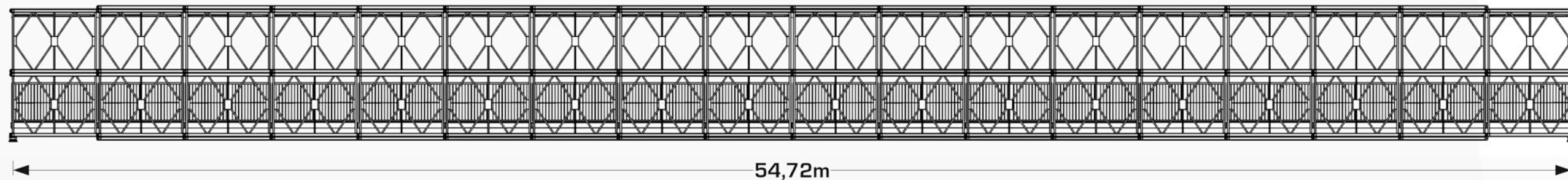
Seitenansicht
