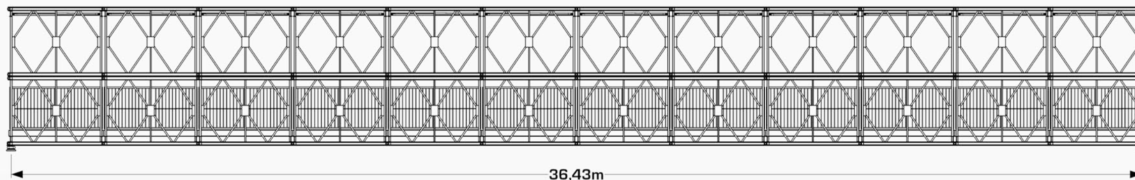
Seitenansicht
