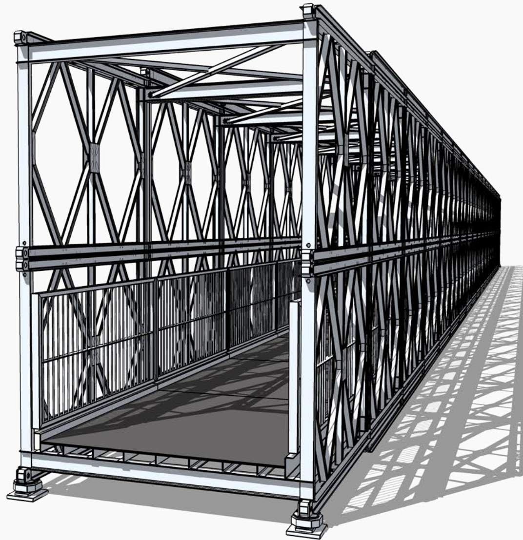
3D-Darstellung
