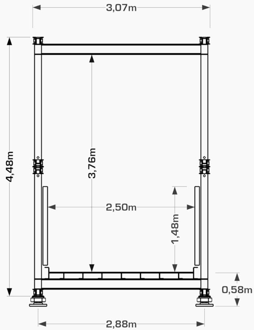
Vorderansicht
