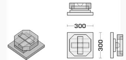
Detail: Lagerplatte
