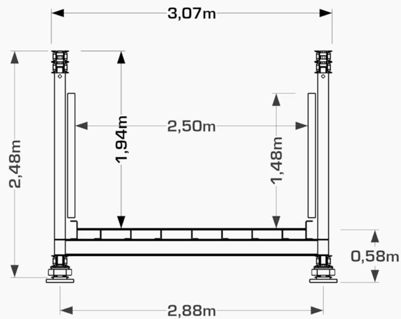
Vorderansicht
