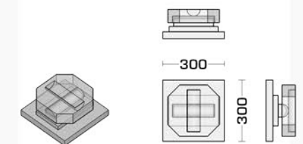
Detail: Lagerplatte
