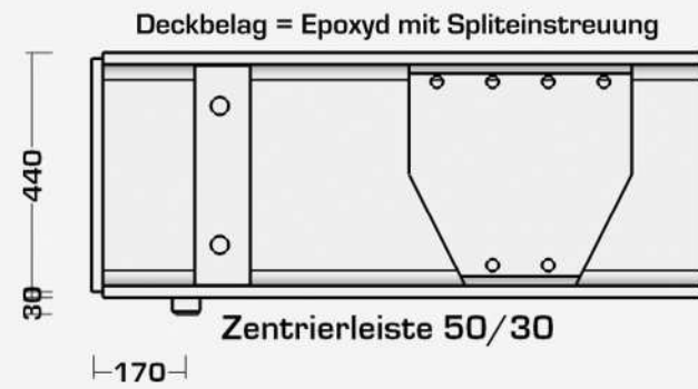
Detail: Auflager
