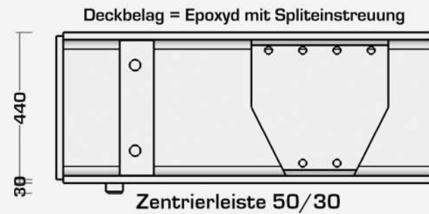
Detail: Auflager
