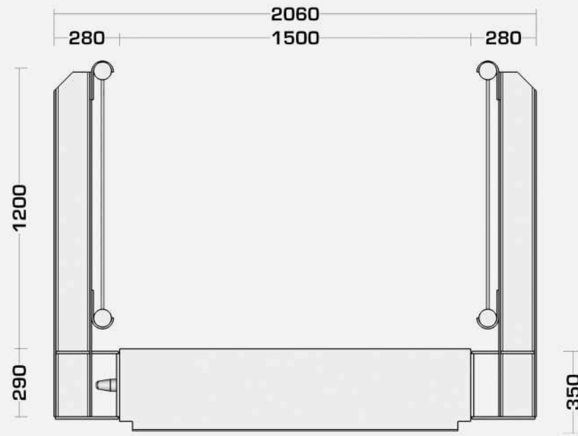
Vorderansicht
