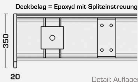
Detail: Auflager
