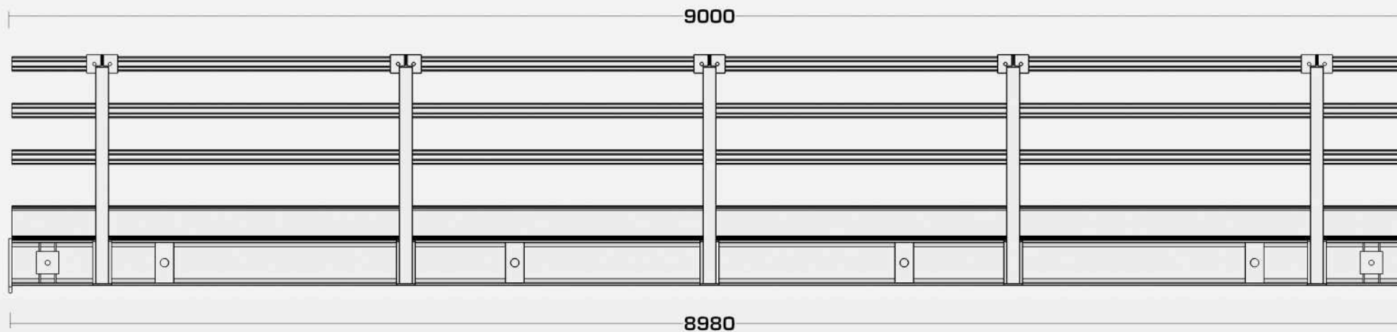
Seitenansicht
