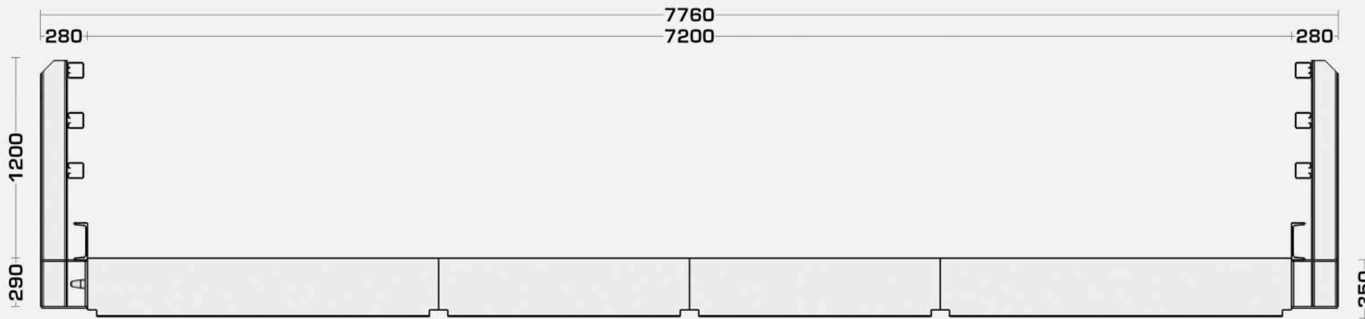
Vorderansicht
