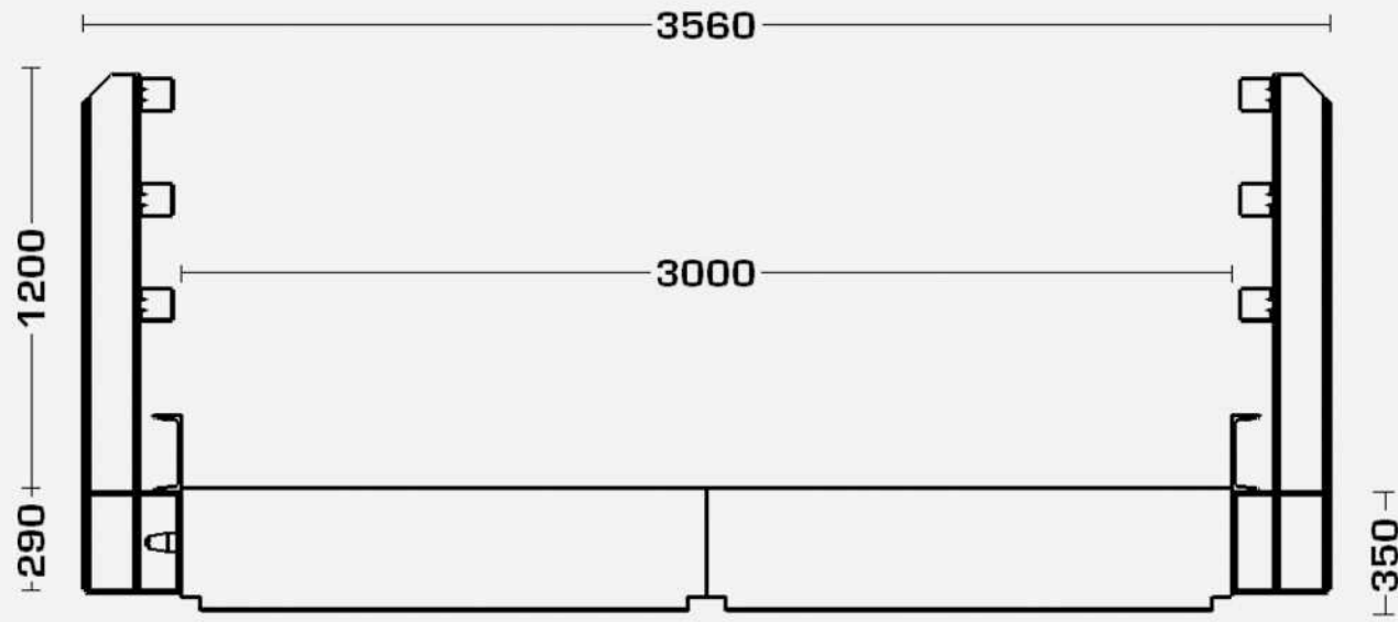
Vorderansicht
