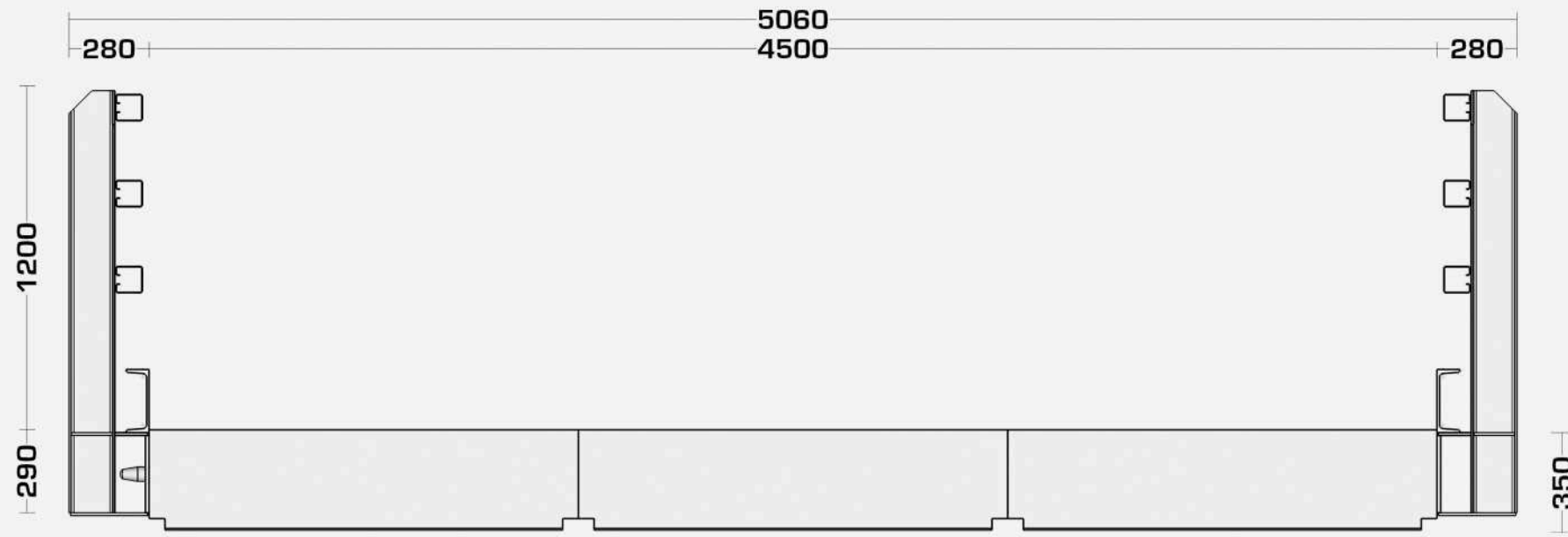
Vorderansicht
