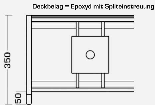
Detail: Auflager
