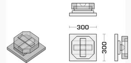
Detail: Lagerplatte
