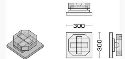
Detail: Lagerplatte
