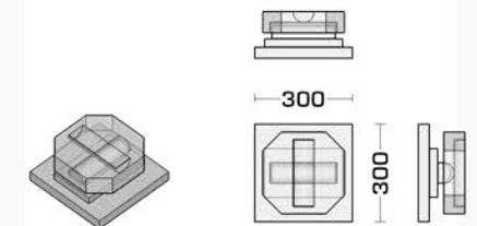
Detail: Lagerplatte
