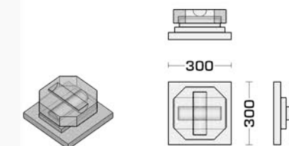
Detail: Lagerplatte
